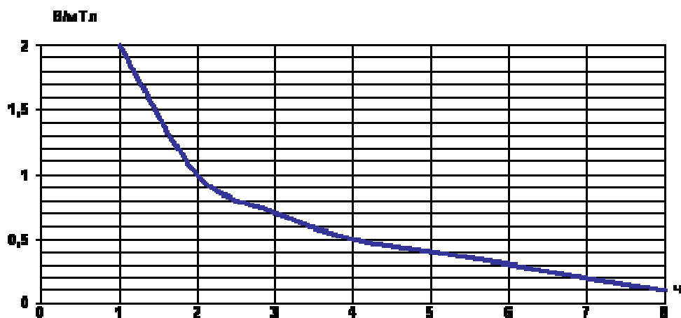
КРИВАЯ ИНТЕРПОЛЯЦИИ ПДУ МАГНИТНЫХ ПОЛЕЙ ЧАСТОТ 50 Гц В ЗАВИСИМОСТИ ОТ ВРЕМЕНИ
